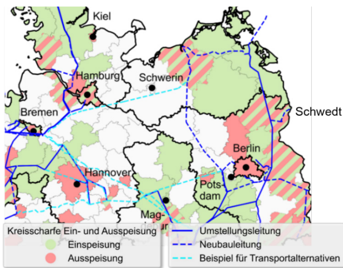
Abbildung 8: Aktueller Planungsstand des Wasserstoff-Kernetzes Quelle: Ferngas Netzgesellschaft mbH (2023): Aktueller Planungsstand Wasserstoff-Kernetz, https://www.ferngas.de/aktueller-planungsstand-wasserstoff-kernetz/ , letzter Zugriff: 05.08.2024.
