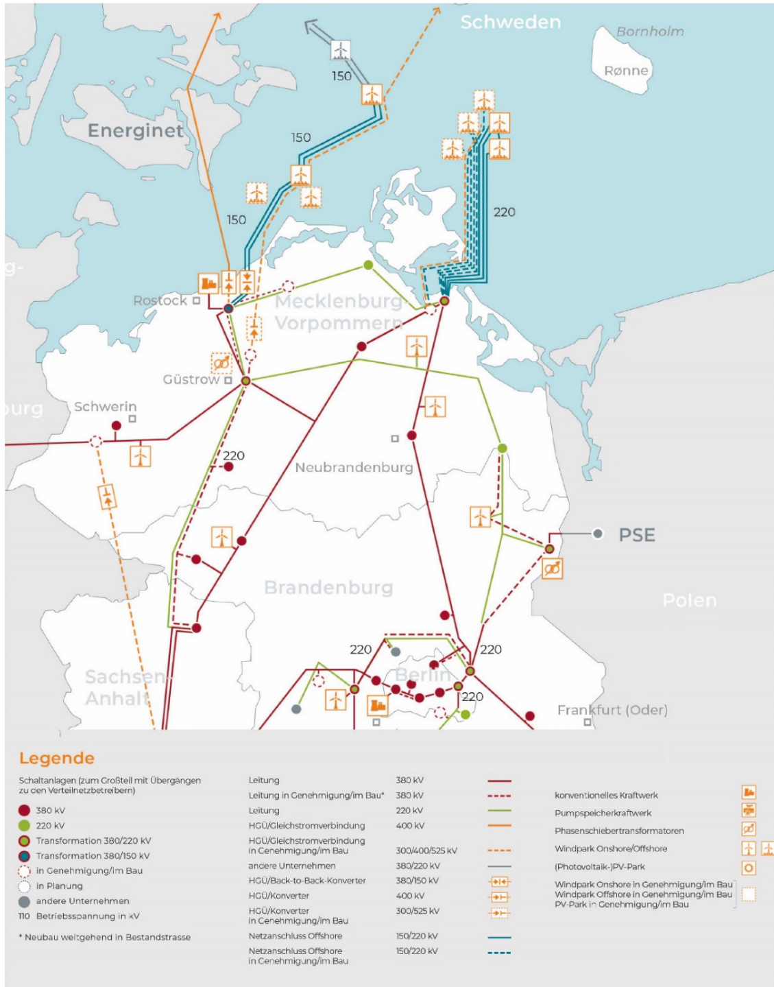
Abbildung 9: Verlauf der Höchstspannungleitung Quelle: 50Hertz Transmission GmbH (Hrsg.) (2023) (Hrsg.): Netzausbau, Stand: Mai 2023; https://www.50hertz.com/ , letzter Zugriff: 20.05.2024.
